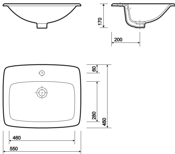
E100 550 1TH countertop basin
