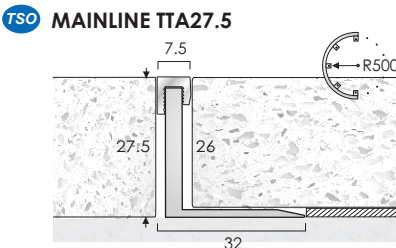
TSO MAINLINE TTA27.5
