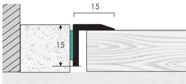
PTP 15/15 OSF
