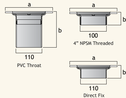
Solid Plate Grate + Bezel
