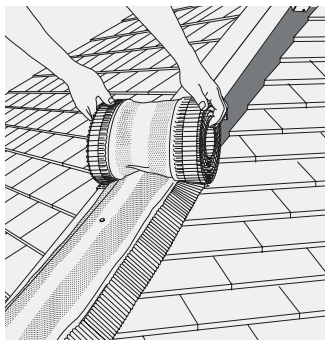
Fig. 58 – Roll out HipFast roll
