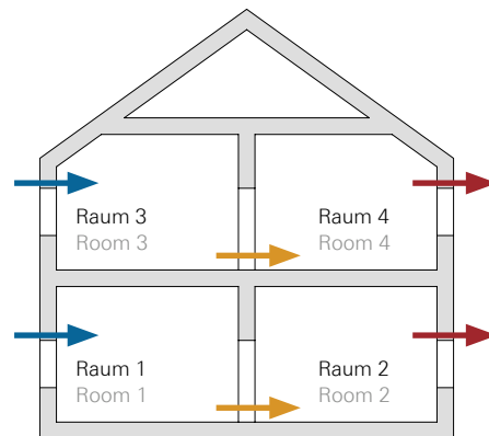
Beispiel 1 Querlüftung mit Außenluftdurchlässen Example 1 Cross ventilation with external air openings
