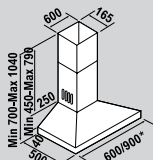
60 Chimney
