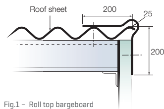
Fig.1 – Roll top bargeboard
