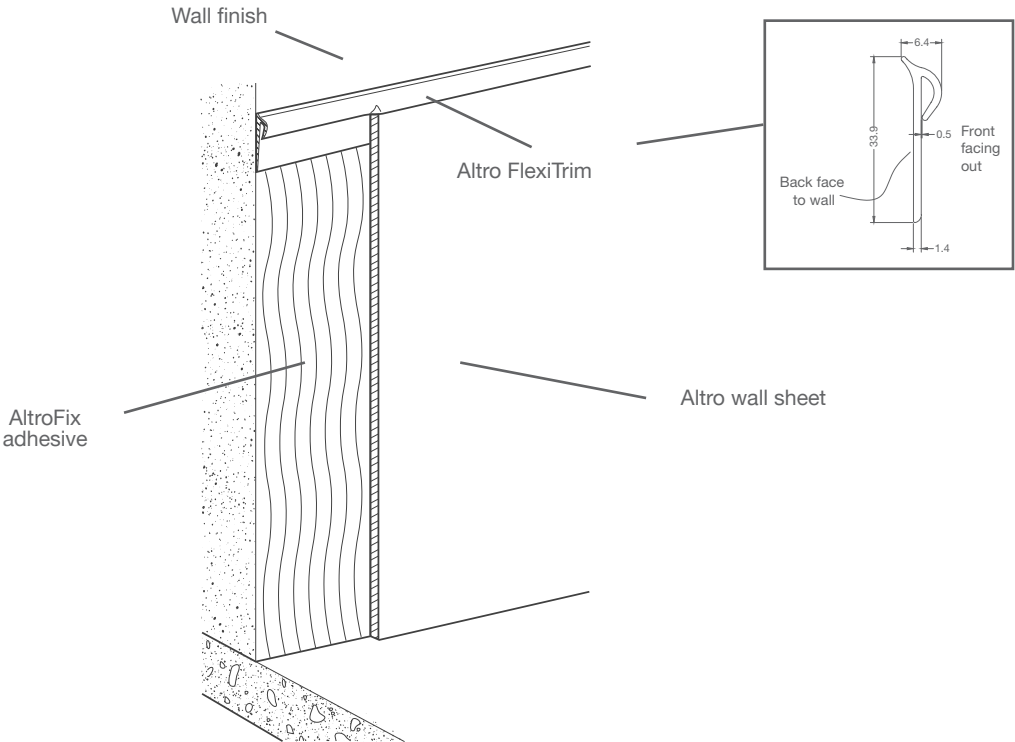
Altro wall sheet at dado height with Altro FlexiTrim
